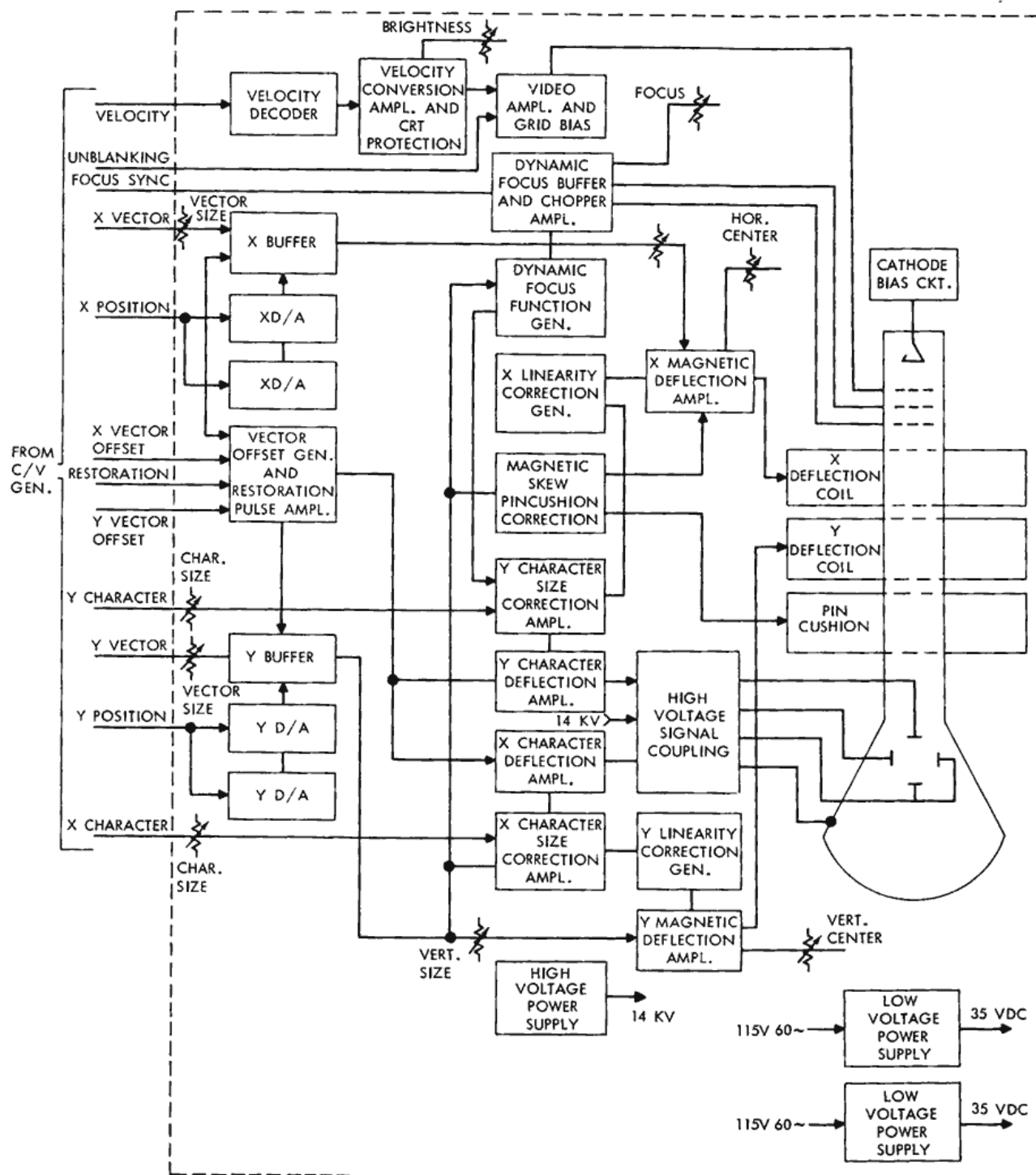
Figure 4—Digital display.
